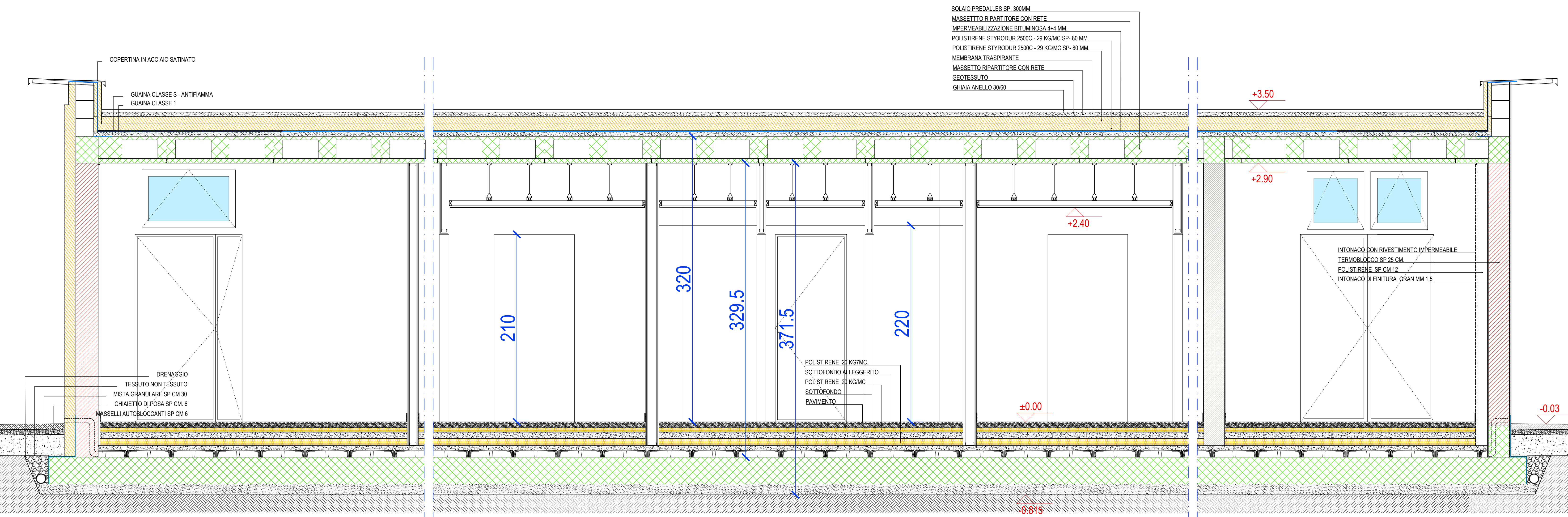
SEZIONE EE
