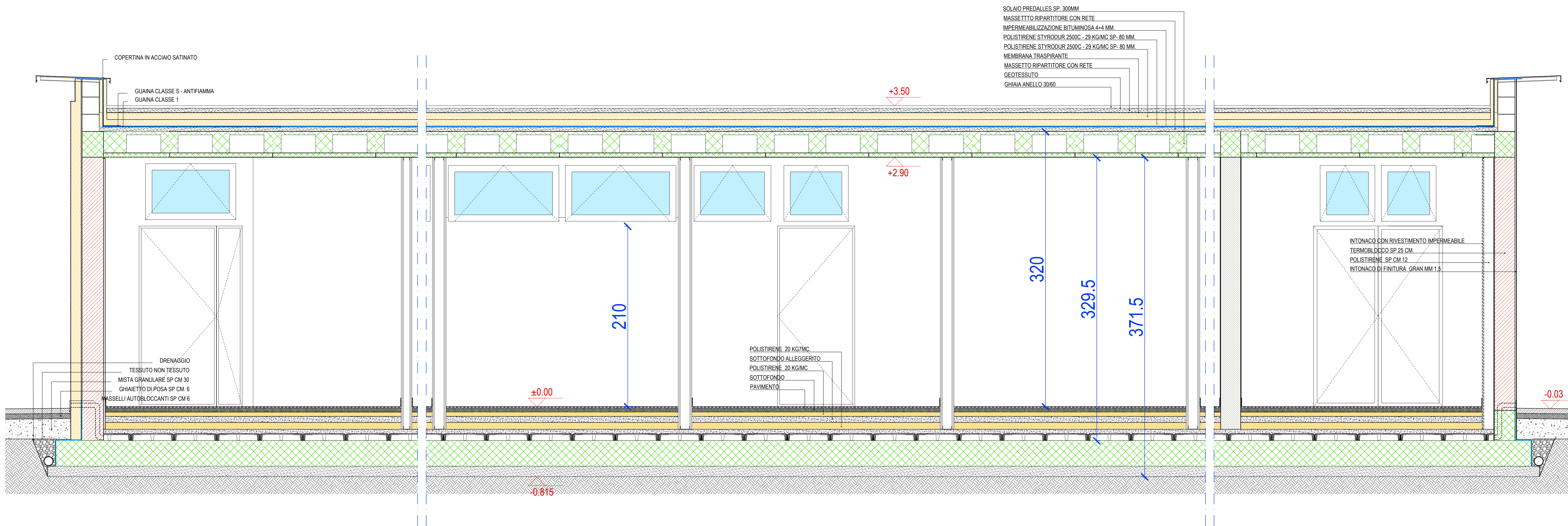
SEZIONE DD
